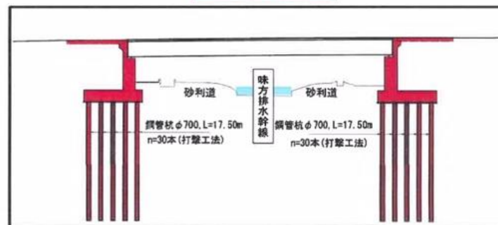
工事箇所 側面図
