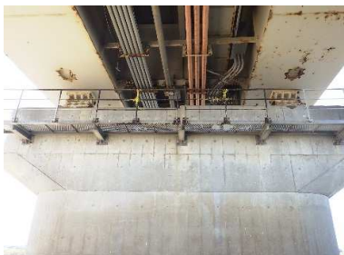
大河津橋の現在の点検通路
