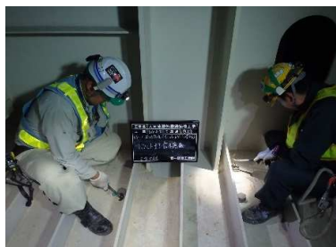
橋のボルトの緩み調査
