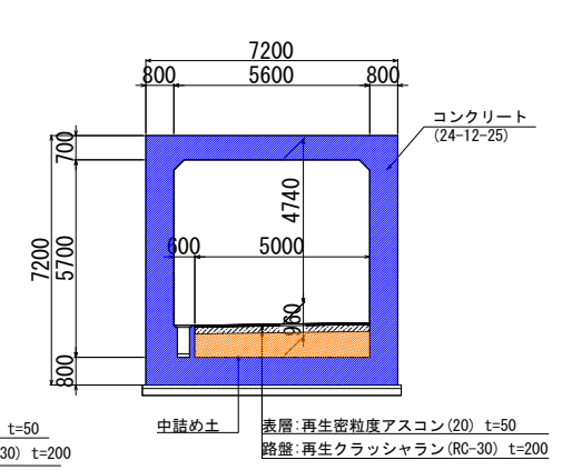
(5号横断函渠)
