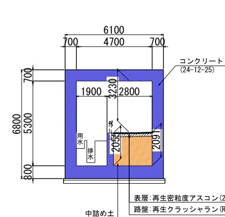
(4号横断函渠)
