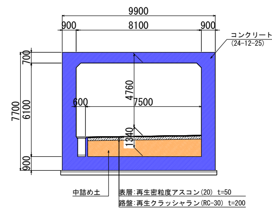
(3号横断函渠)
