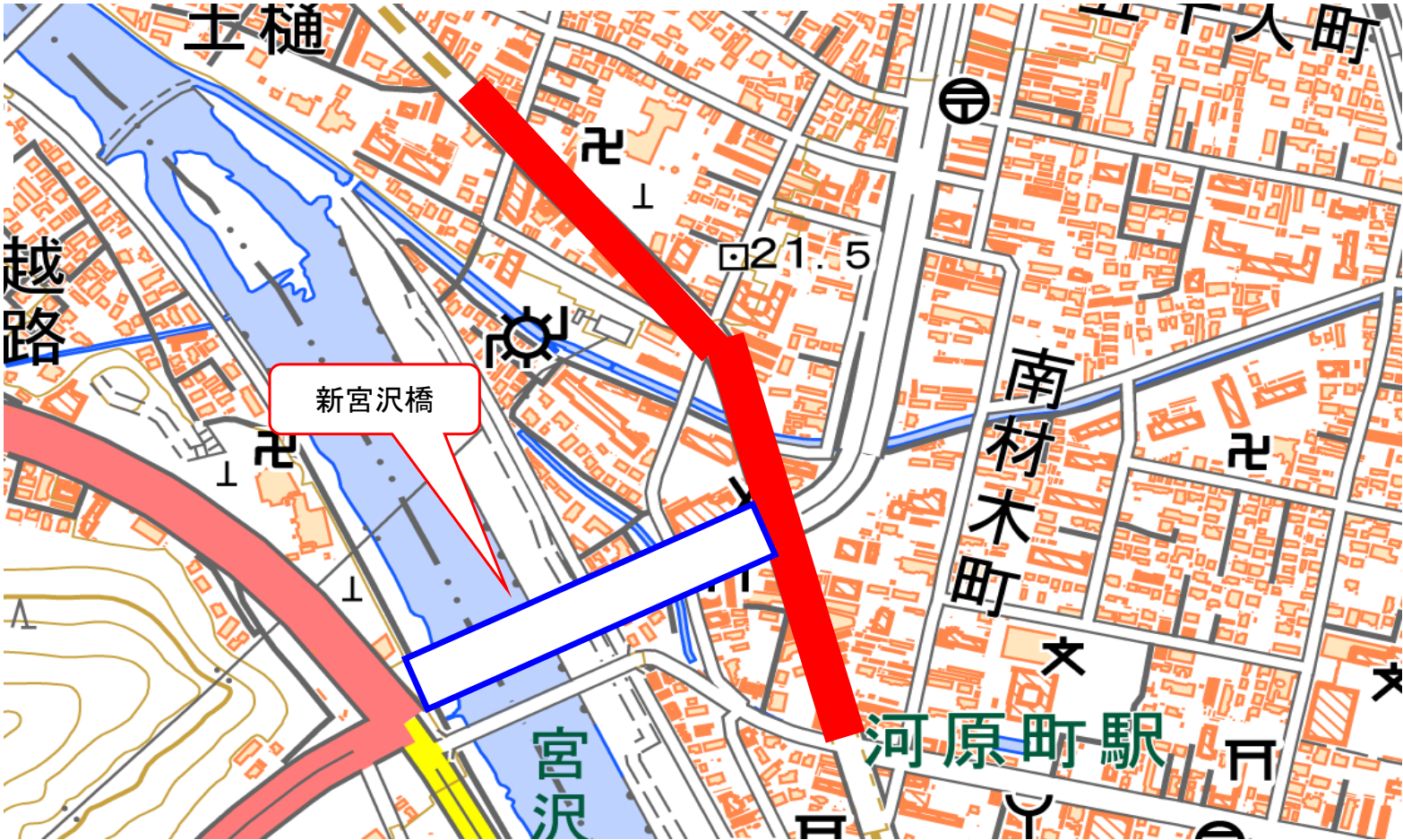
赤:路面切削施工範囲
