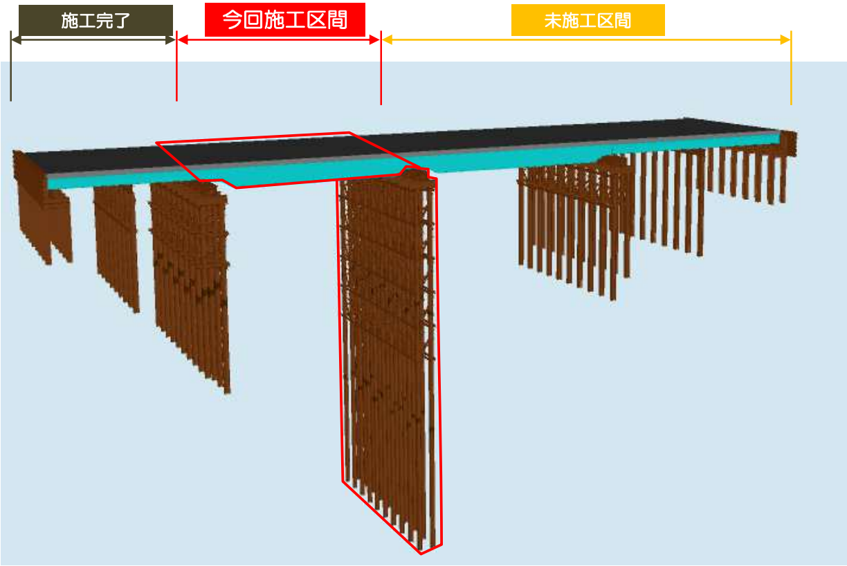
〔側面図〕
